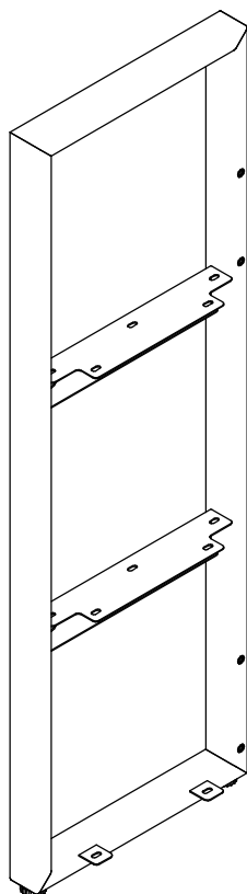
A-112.11.1140 Опора боковая 50x25 для стеллажа h=1140 (Левая)
